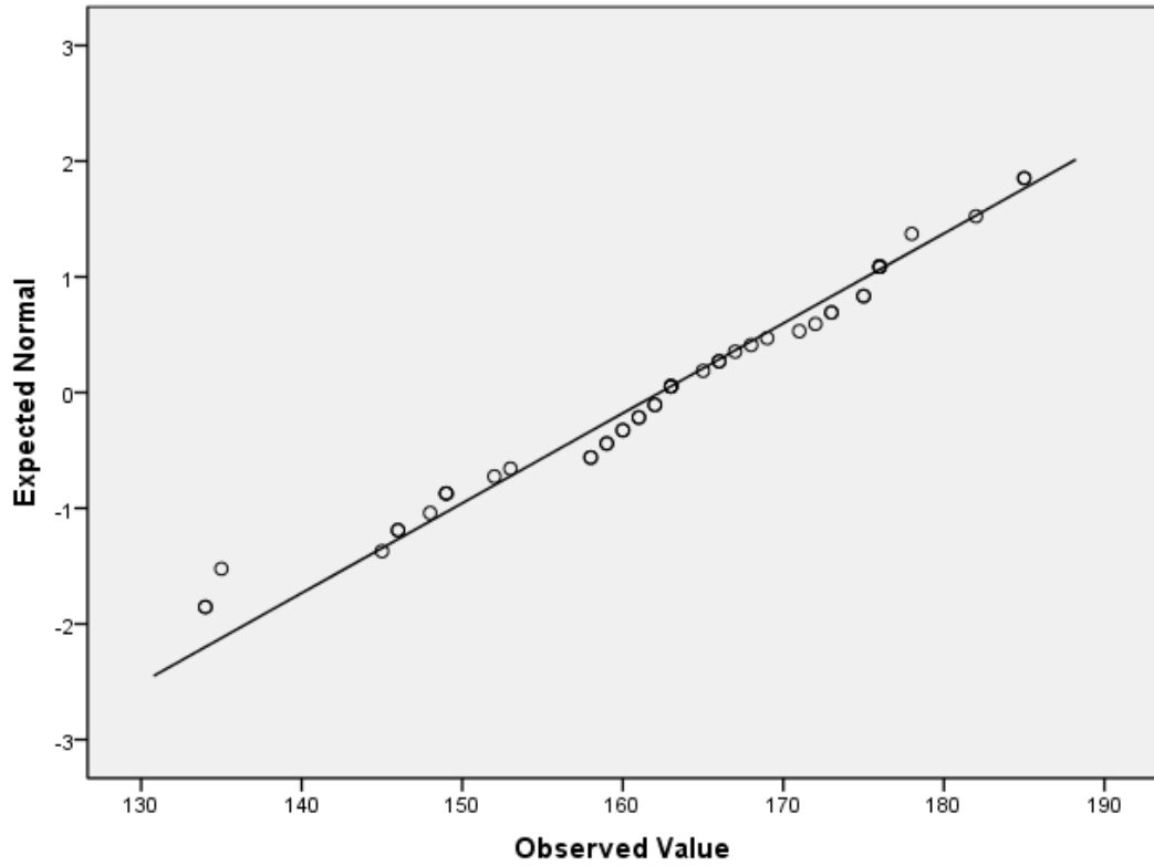
Normal Q-Q Plot of KEPUASAN KERJA
