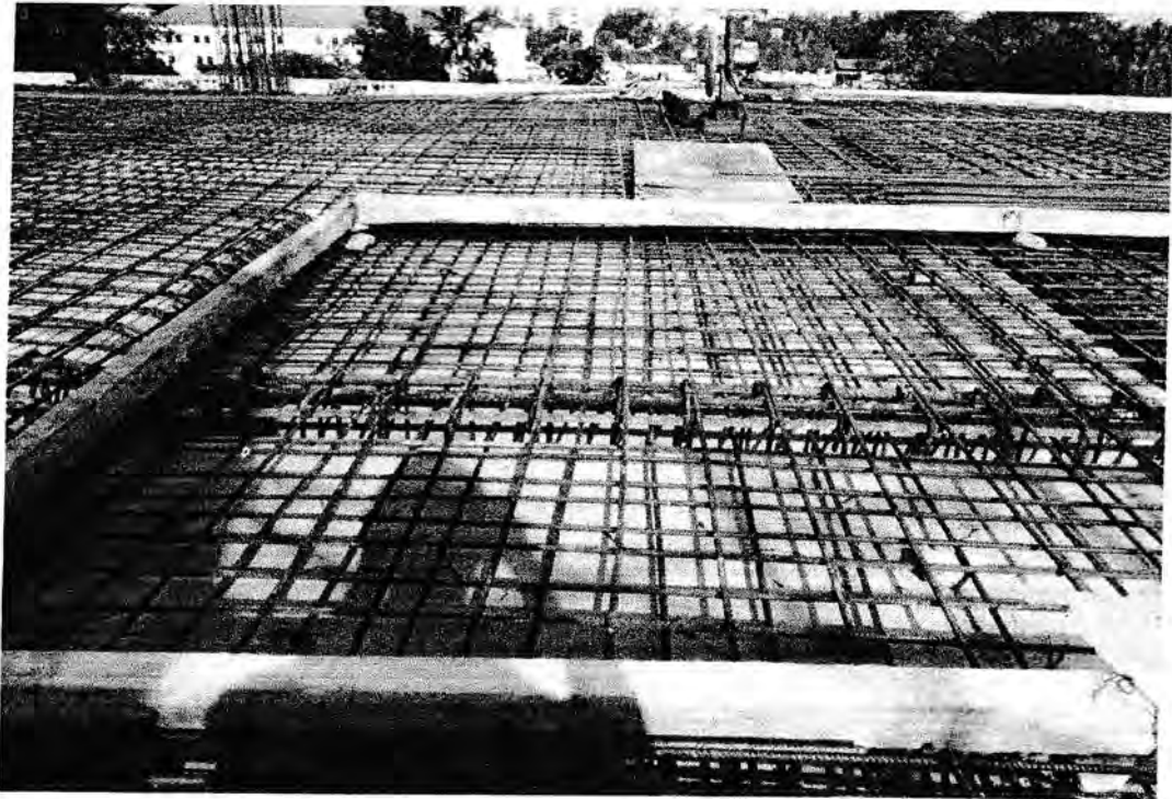
Gambar. Plat tulangan plat lantai yang sudah jadi Lokasi : komplek asrama haji medan
