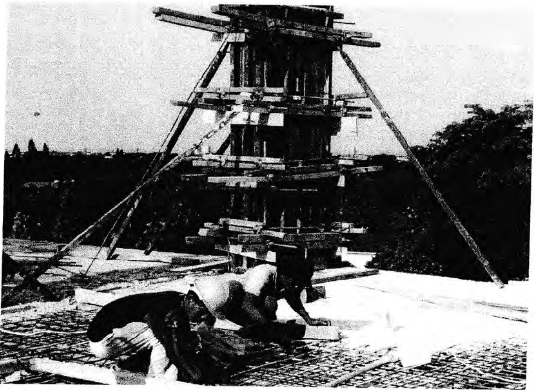
Gambar. Proses Pengeringan Kolom Lokasi : komplek asrama haji medan
