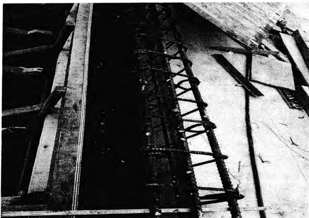
Gambar bekisting pada balok Lokasi : komplek asrama haji medan
