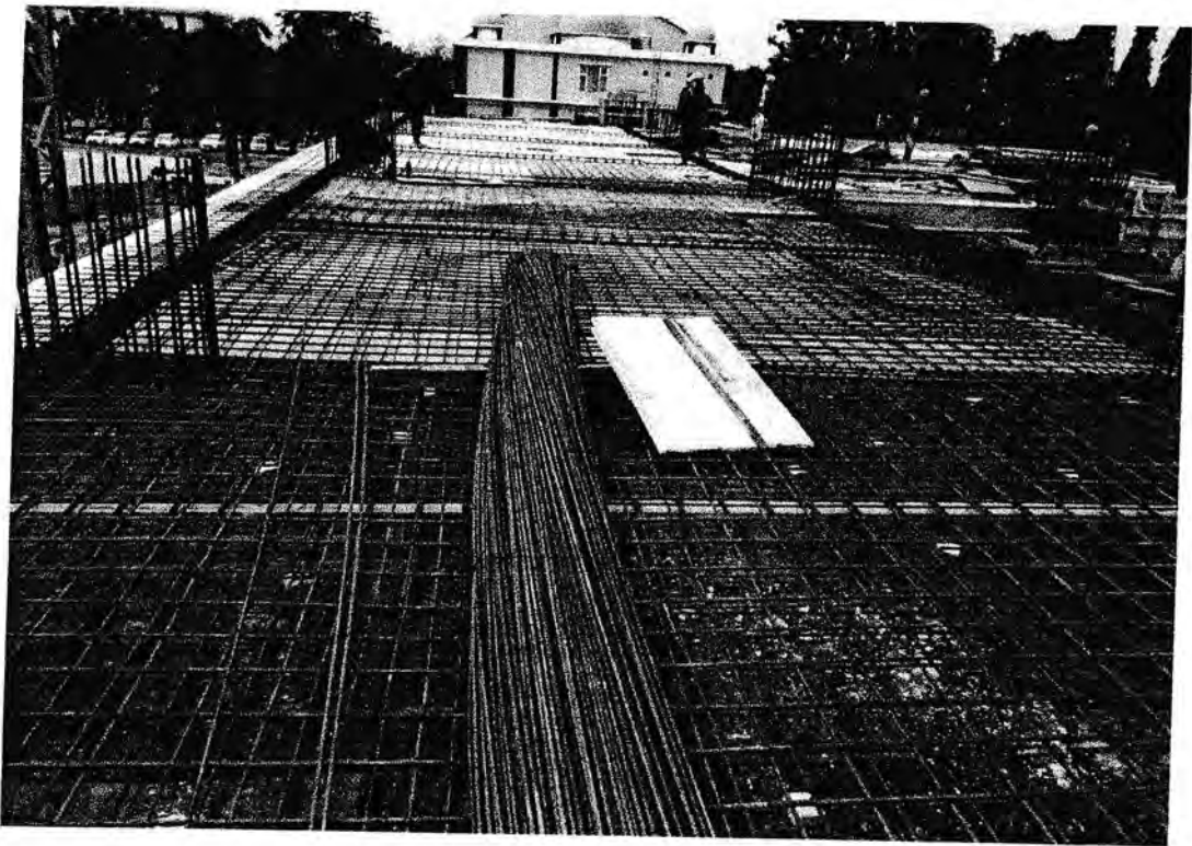
Gambar 3.10 Pembesian Plat Lantai
