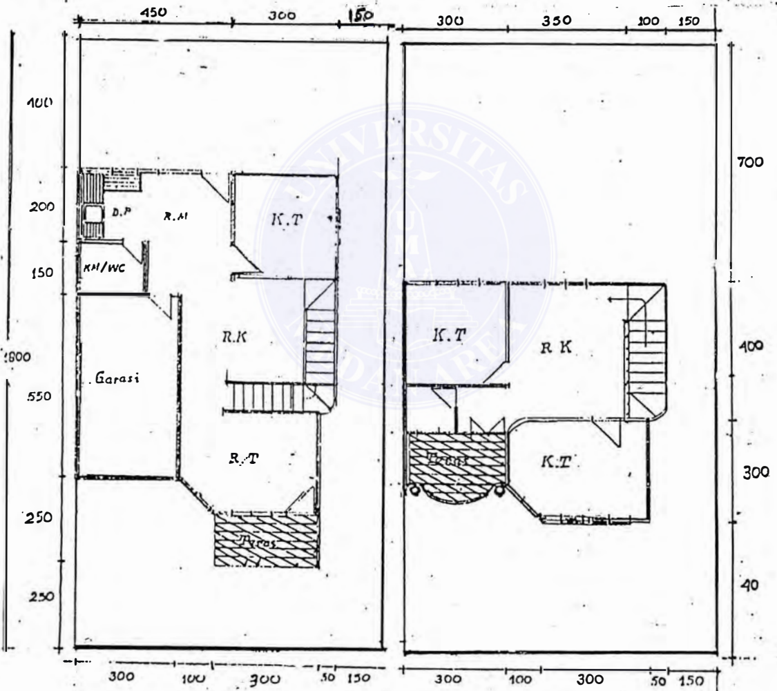
Lantai I 1 : 100
