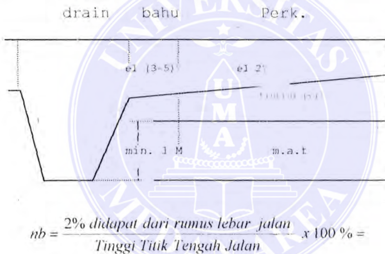
Gambar II.4. Sistem pembuangan air pada jalan Sumber : Teknik Pemeliharaan Jalan
