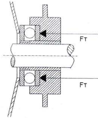
Gambar 10. 4. Bantalan Pembebas
