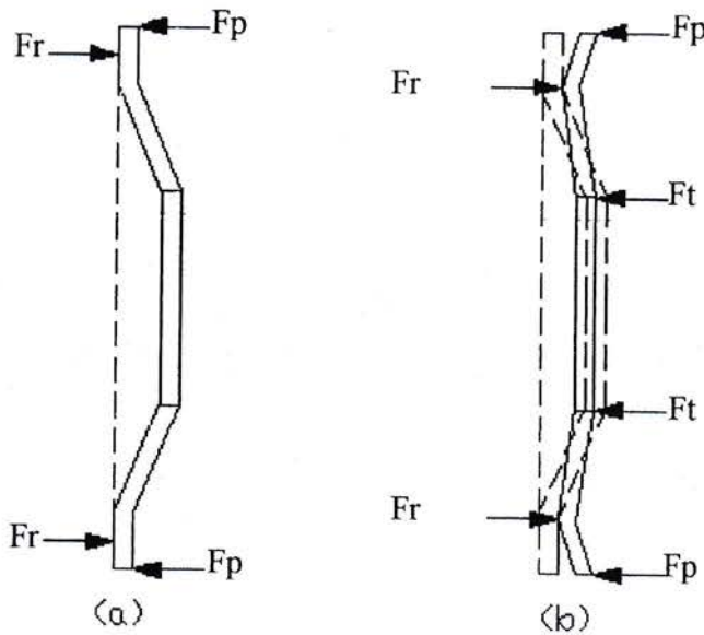
Gambar 8. 2. Diagram gaya-gaya yang bekerja pada pegas
