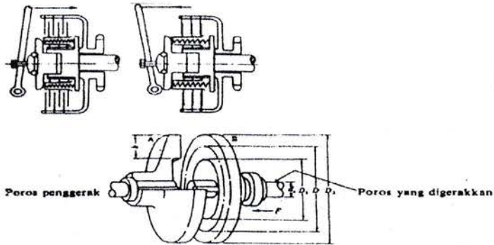
Gambar 2.12. Kopling Plat
