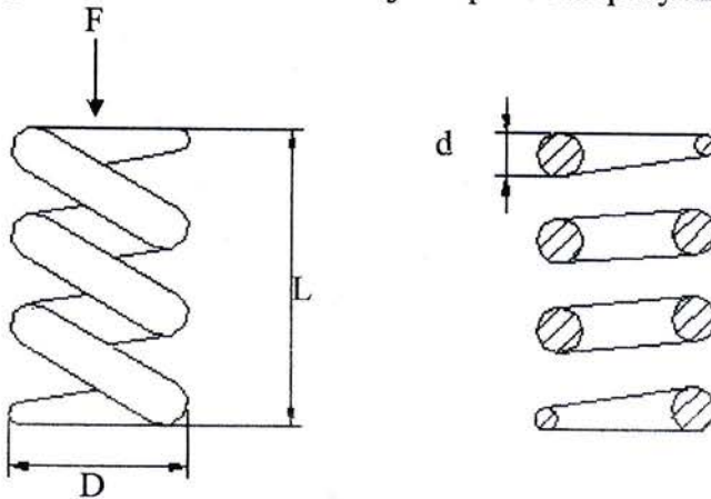
Gambar 8. 3. Pegas Kejut
