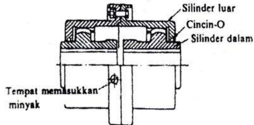
Gambar 2.7. Kopling Gigi
