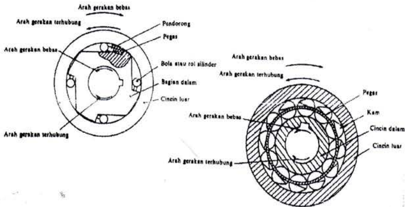
Gambar 2.13. Kopling Friwil
