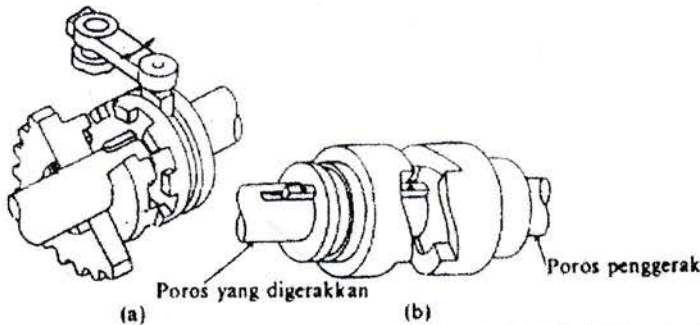
Gambar 2.10. Kopling Cakar
