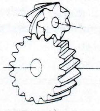
A. Roda gigi miring silang.
