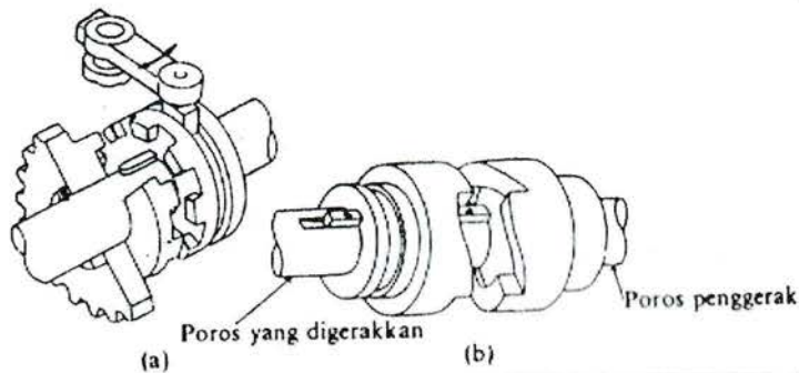
Gambar 2.10. Kopling Cakar
