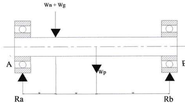
Gambar 10.2. Analisa Gaya Pada Bantalan Pendukung Poros
