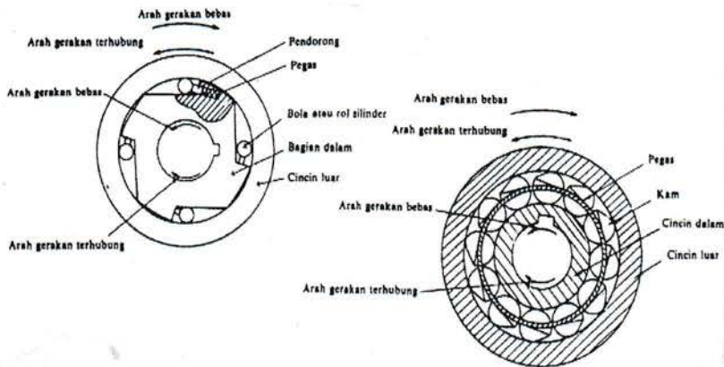
Gambar 2.13. Kopling Friwil
