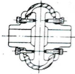
Gambar 2.5. Kopling Karet Ban
