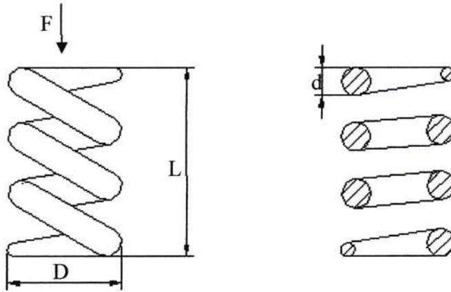
Gambar 8. 3. Pegas Kejut
