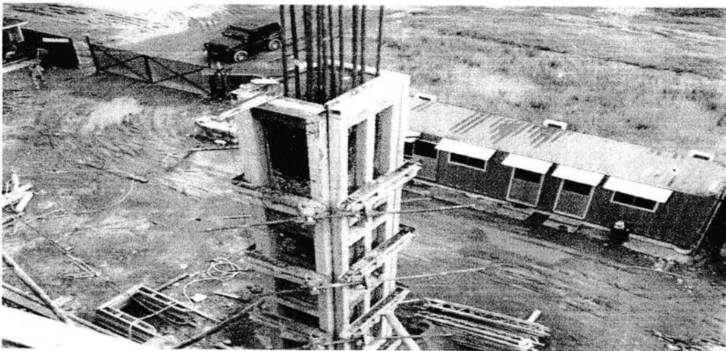
Pemasangan Bekisting Kolom
