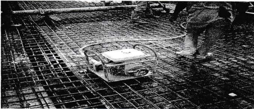
Gambar 2.3 Mesin Vibrator
