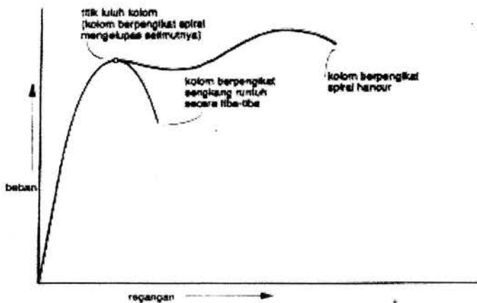
Gambar : Hubungan beban – regangan pada kolom
