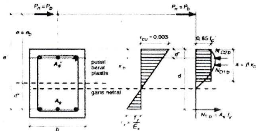
Gambar : Keadaan keseimbangan regangan – penampang kolom persegi
