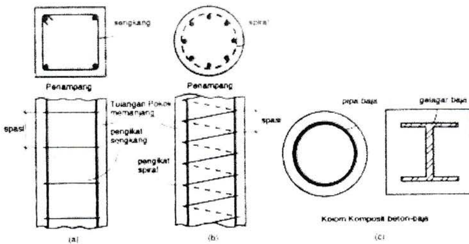
Gambar : Jenis-jenis kolom
