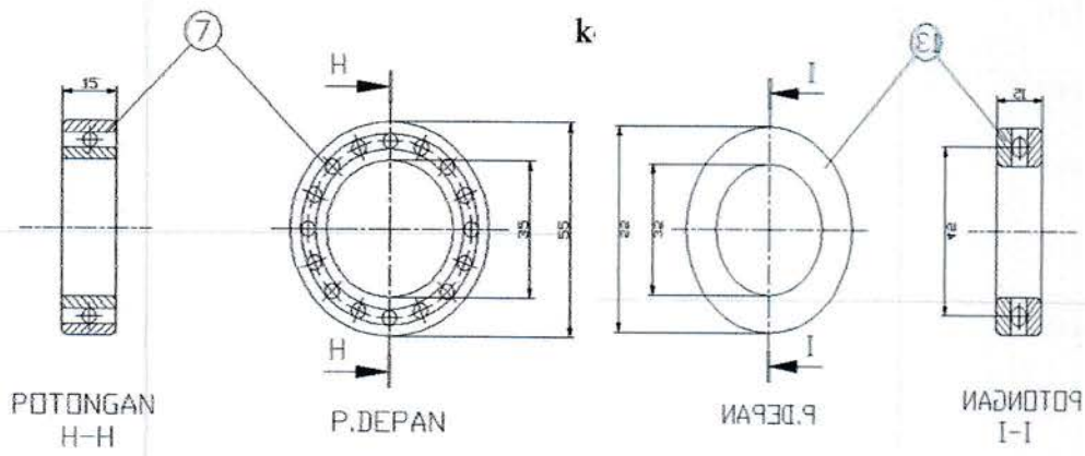
Gambar 3.6 Bantalan Radial (kiri) dan Bantalan Aksial (kanan)
