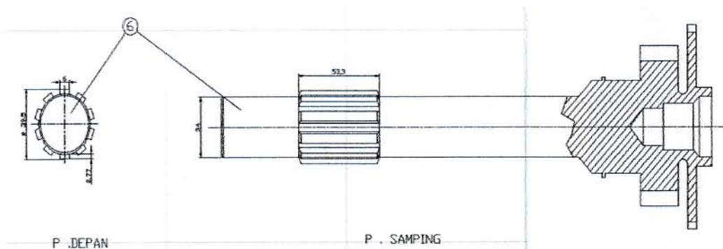
Gambar 3.1 Poros
