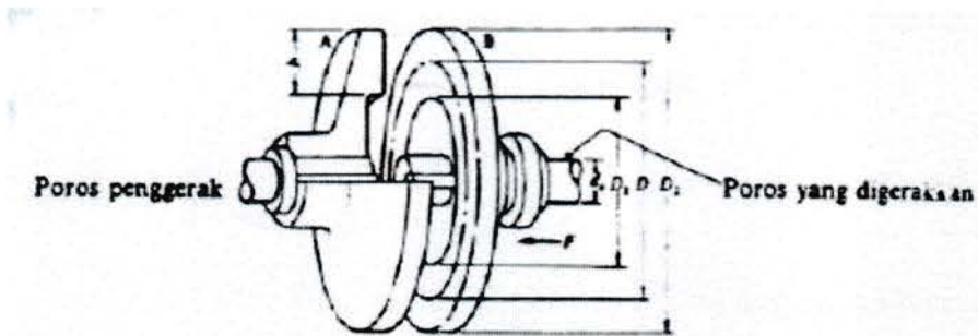
Gambar 2.11 Kopling Plat Tunggal
