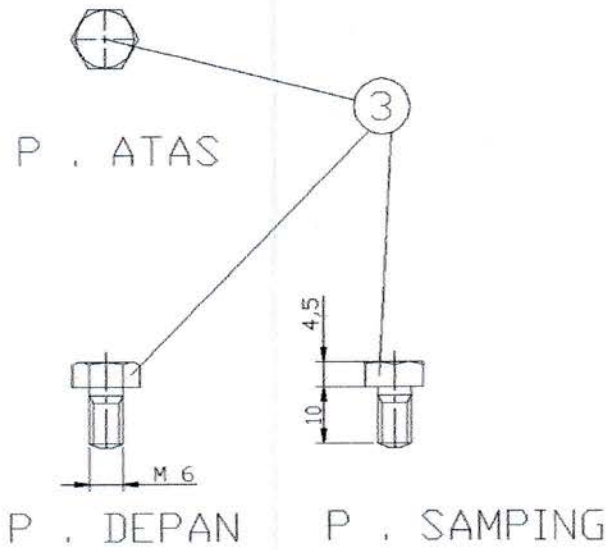
Gambar 3.7 Baut
