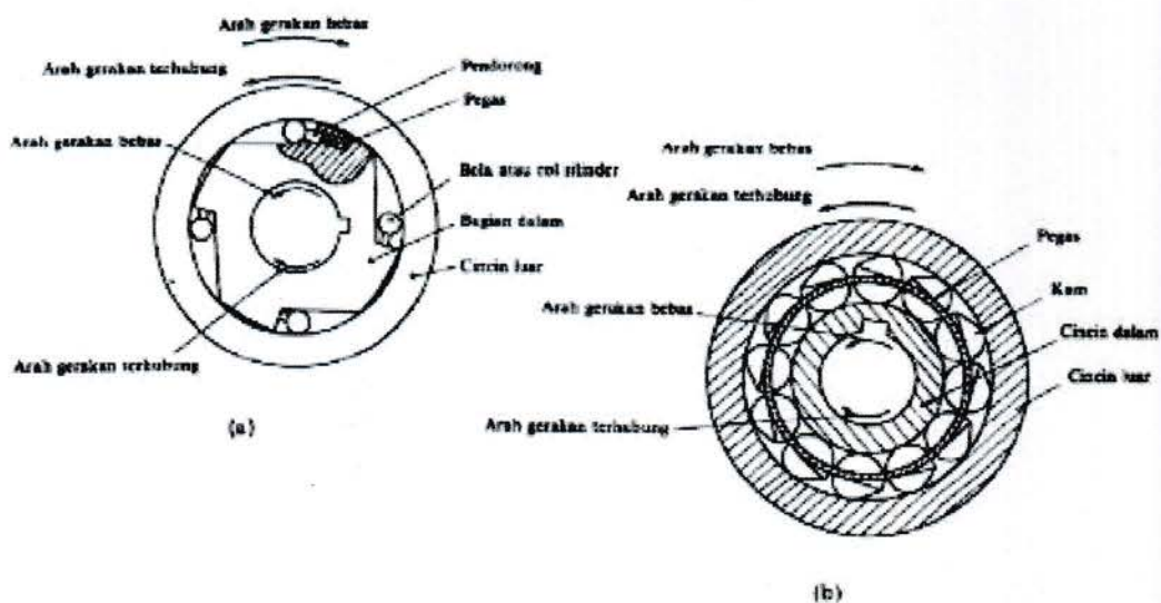
Gambar 2.14 Kopling Friwil
