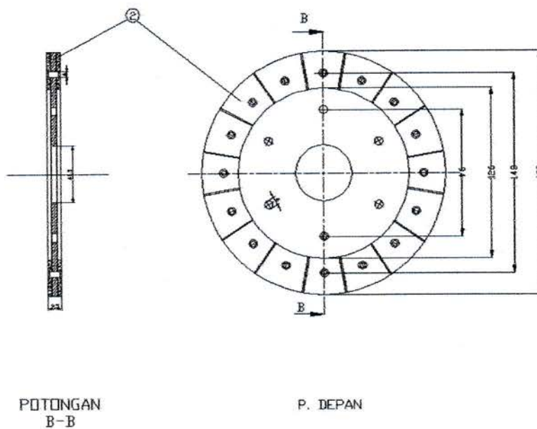
Gambar 3.4 Plat Gesek
