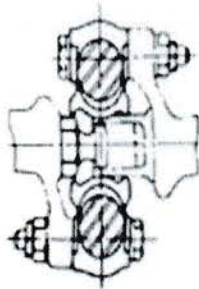
Gambar 2.6 Kopling Karet Bintang
