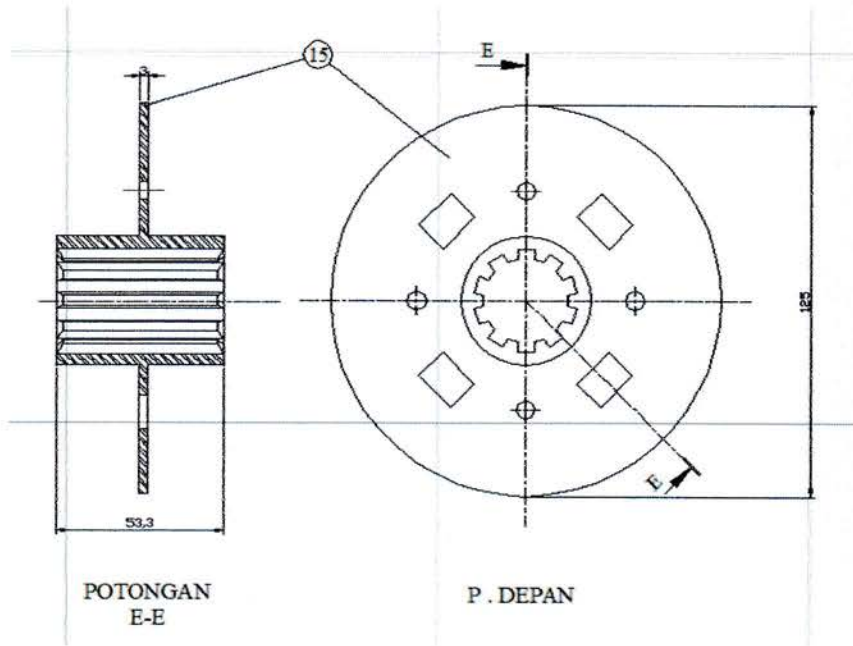
Gambar 3.3 Naaf
