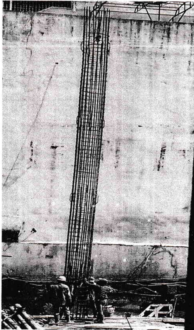
Gambar 4.6 Tulangan di lapangan
