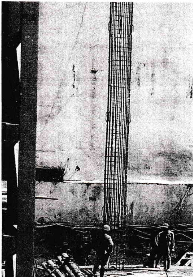
Gambar 3.25 Pekerjaan Pembesian
