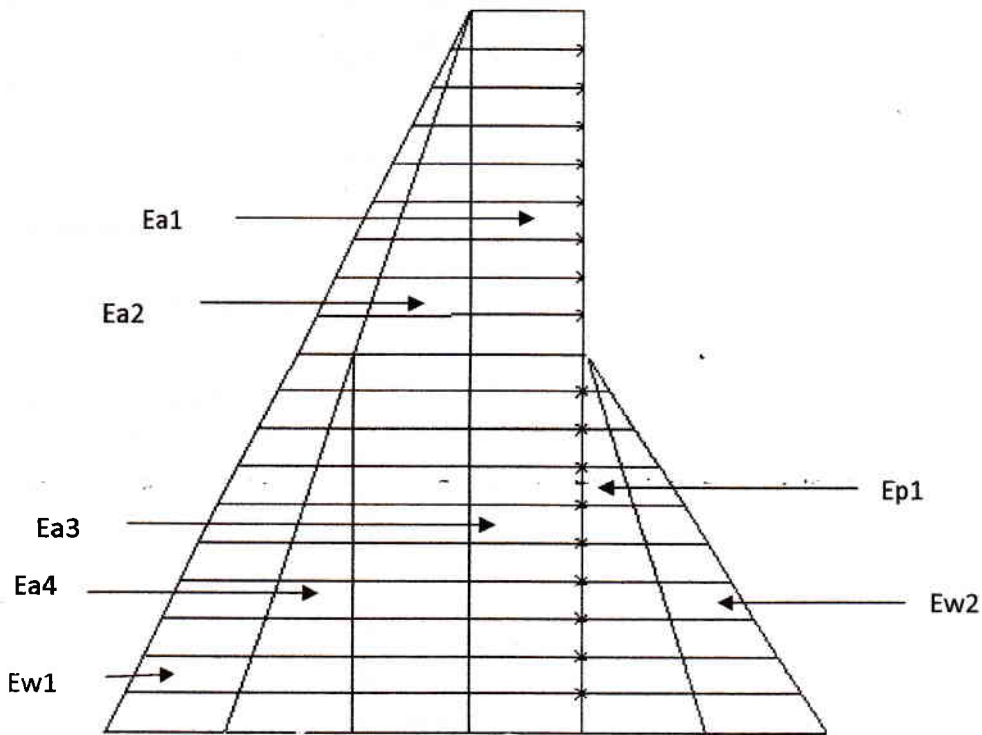
Gambar 4.4 Tekanan Tanah
