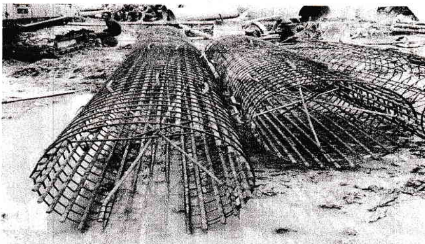
Gambar 3.19 Besi Tulangan
